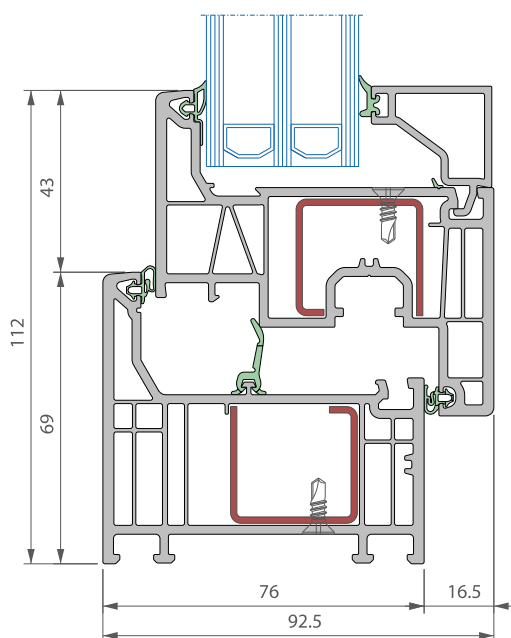
Przekrój pionowy
