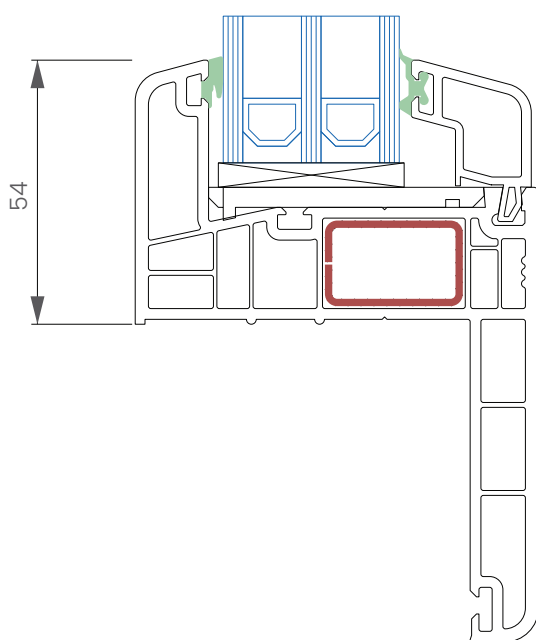
Przekrój pionowy
