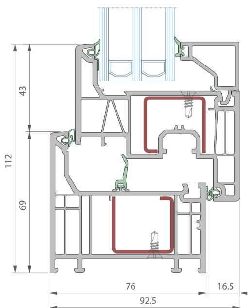
Vertikaler Querschnitt
