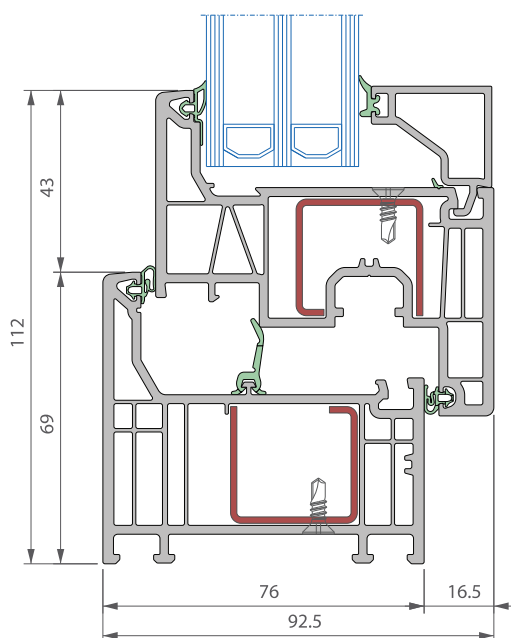
Coupe verticale
